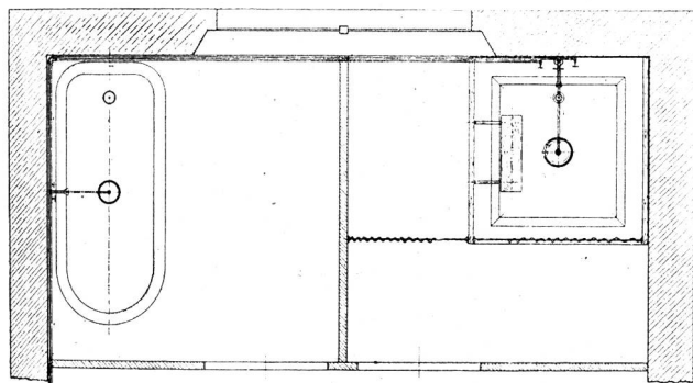
Fig. 1. Grundriß.
