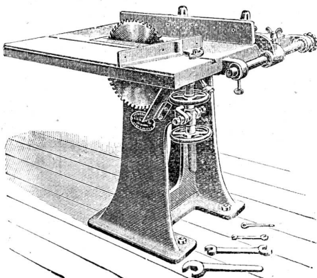
Kreissäge mit Blatt 400 mm zum Nuten u. Falzen eingerichtet.
