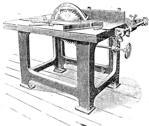
Kreissäge in 3 Grössen für sämtliche Schreinerzwecke passend.
