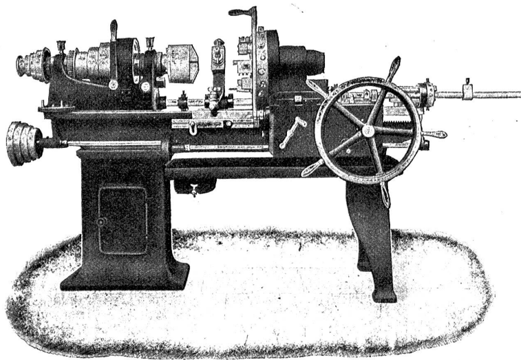
Revolver-Drehbank R 35.
