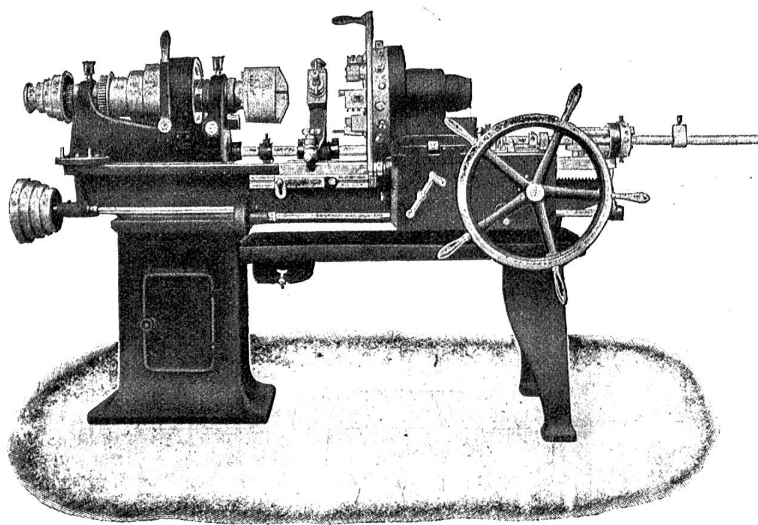
Revolver-Drehbank R 35.
