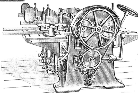
Dreiseitige Hboelmaschine.
