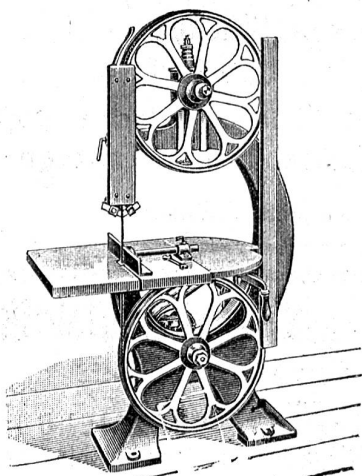
Kleinere Bandsäge.
