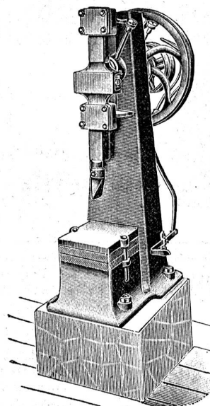
Holzspaltmaschine.
