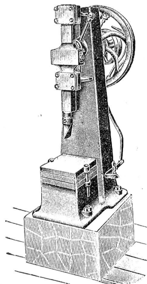
Holzspaltmaschine.
