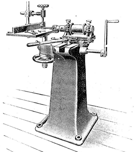
Langlochbohrmaschine.
