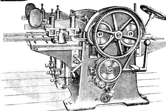
Dreiseitige Hboelmaschine.
