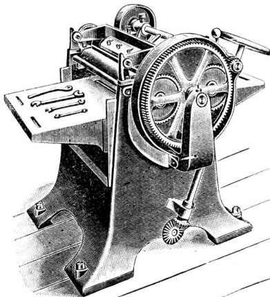
Dickehobelmaschine.
