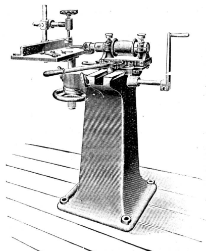
Langlochbohrmaschine.
