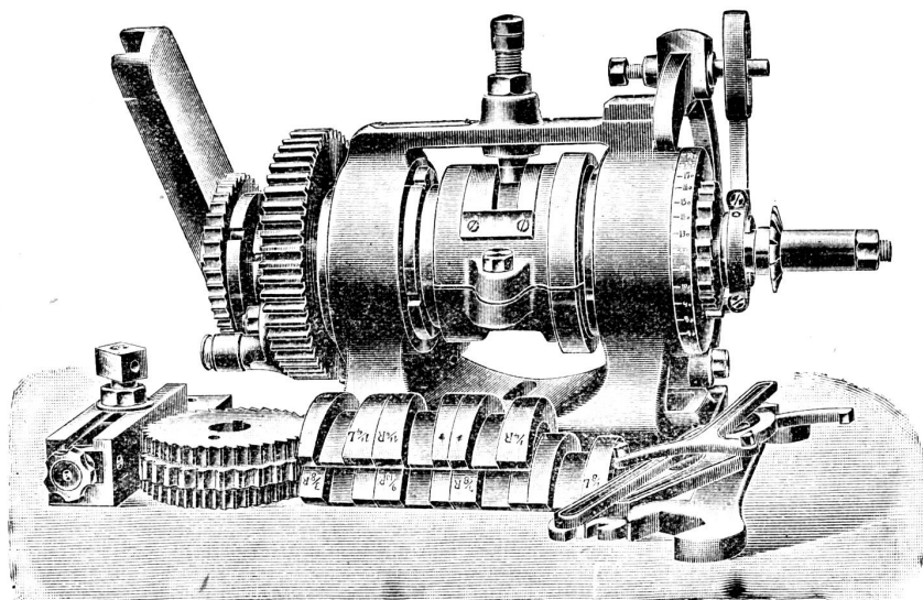
Hinterdreh-Apparat No. 1.
