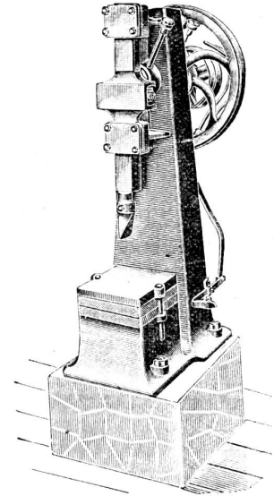
Holzspaltmaschine.
