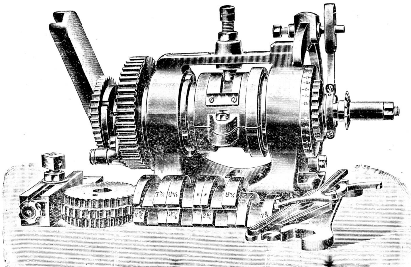
Hinterdreh-Apparat No. 1.
