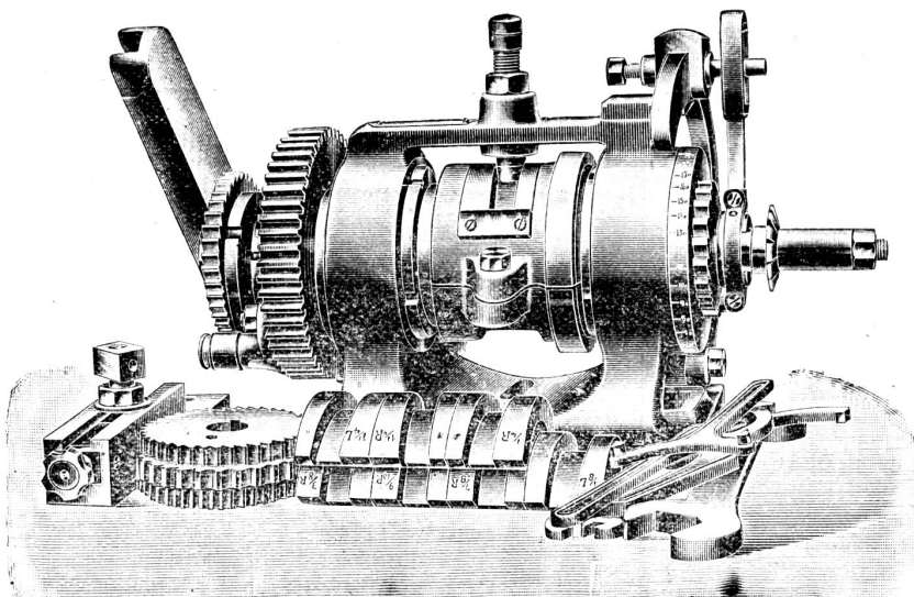
Hinterdreh-Apparat No. 1.
