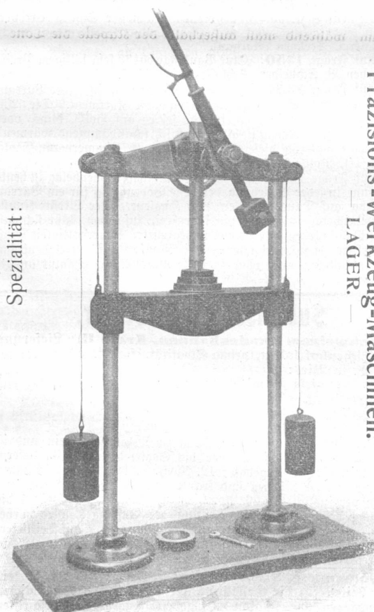
Dorn-Eintreibe-Pressen.
