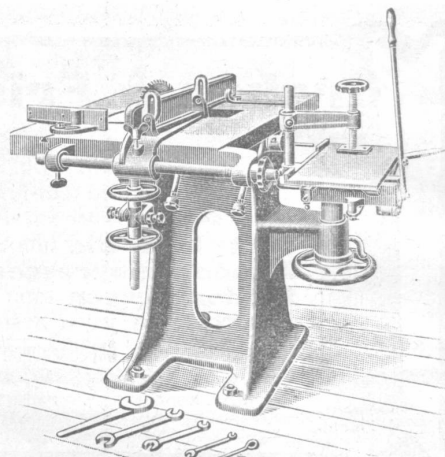
Kreissäge kombiniert mit Langlochbohrmaschine.
