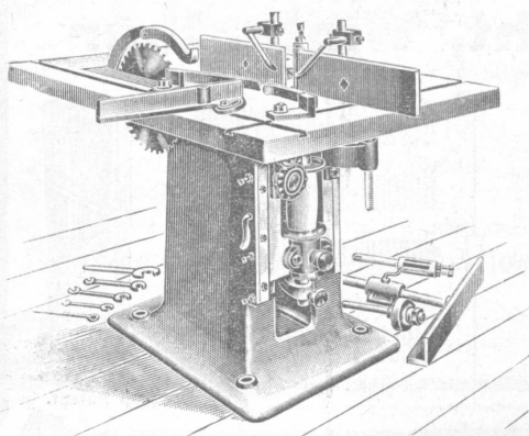
Kreissäge kombiniert mit Kehlmaschine.
