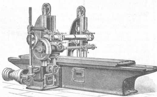
Plan-Fräsmaschine.
