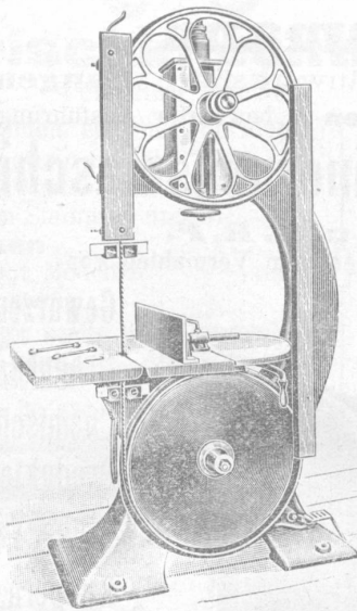
Bandsäge in 5 Grössen.
