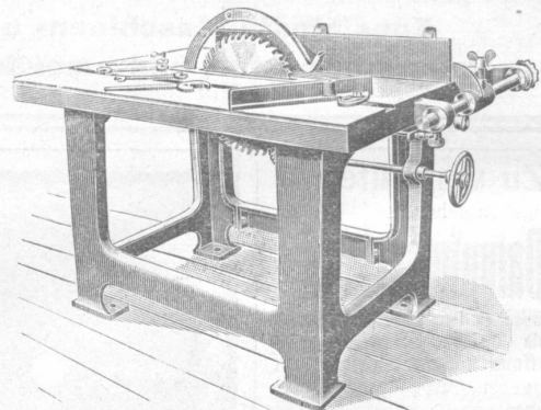
Kreissäge
