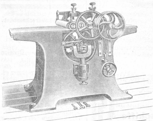
Sandpapierschleifmaschine.
