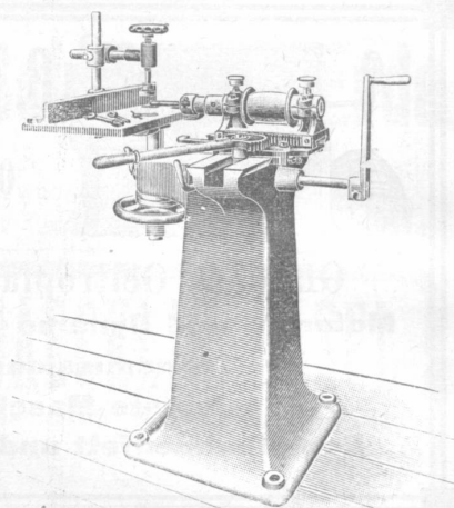
Langlochbohrmaschine.
