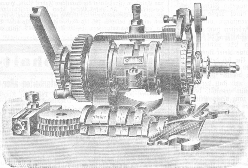
Hinterdreh-Apparat No. 1.
