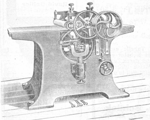
Sandpapierschleifmaschine
