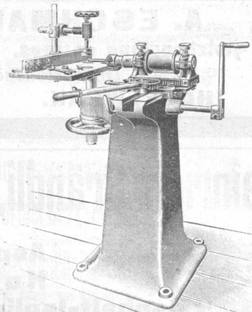
Langlochbohrmaschine.
