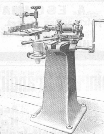
Langlochbohrmaschine.
