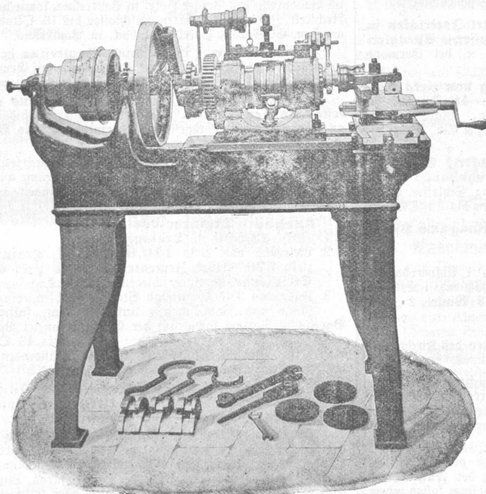
Fräser-Hinter-Drehbank.
