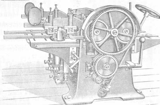
Dreiseitige Hobelmaschine.
