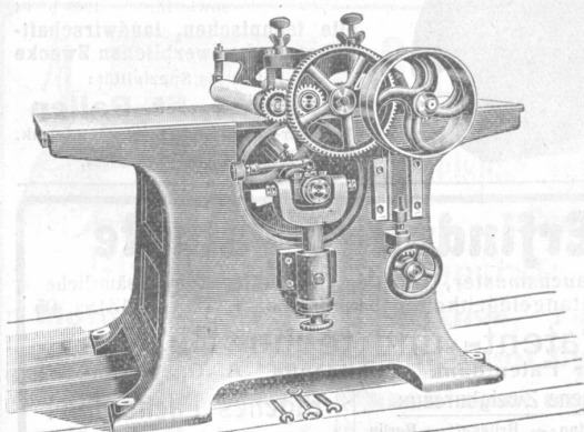
Sandpapierschleifmaschine
