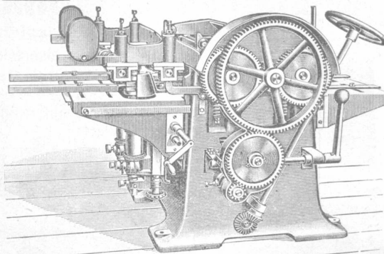
Dreiseitige Hobelmaschine.
