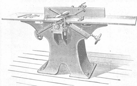
Abrichtmaschine.
