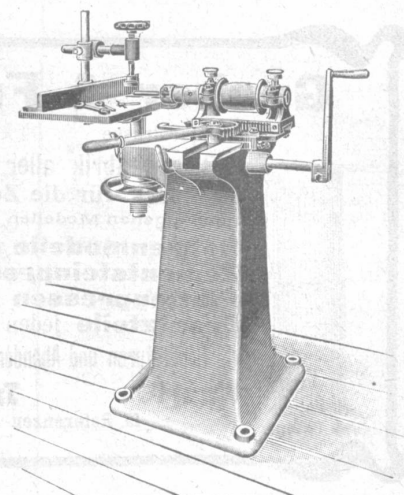
Langlochbohrmaschine.
