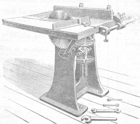
Kreissäge
