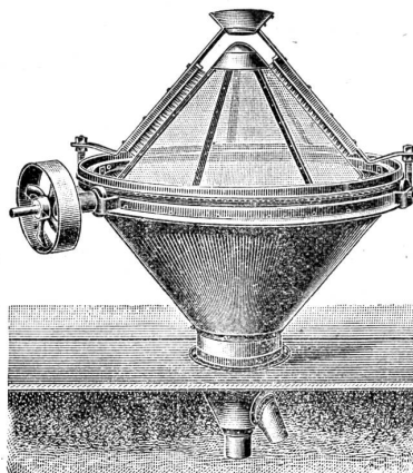
Sichtapparat
