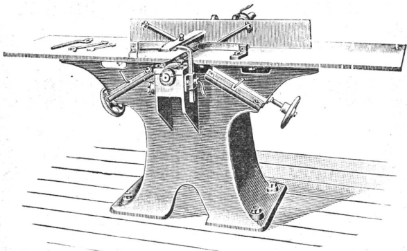
Abrichtmaschine.
