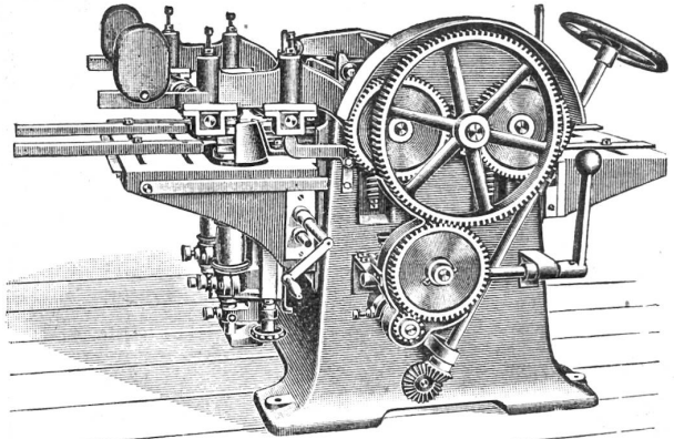
Dreiseitige Hobelmaschine.
