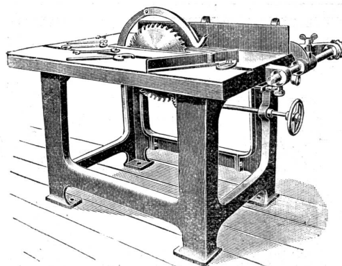
Kreissäge
