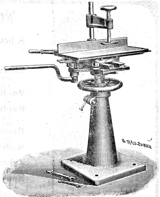
Bohrständer
