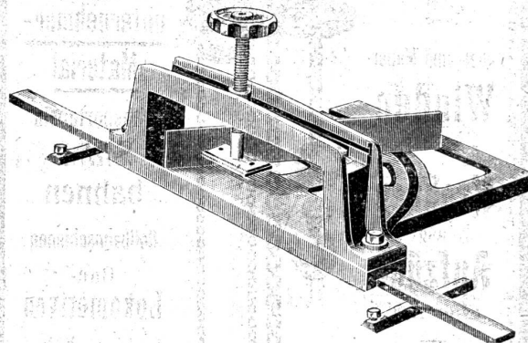
Zapfenschneidtischchen
