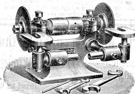
Kehlmesserschleifapparat
