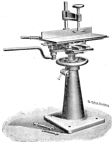
Bohrständler
