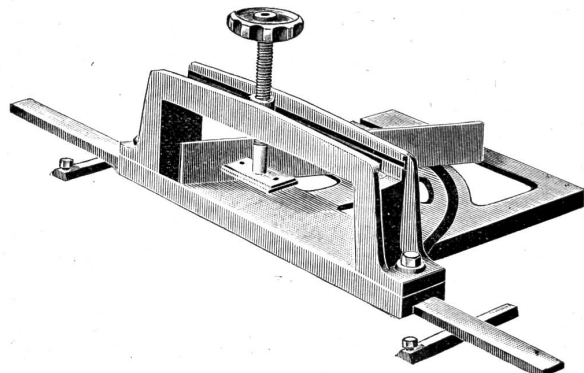
Zapfenschneidtischchen
