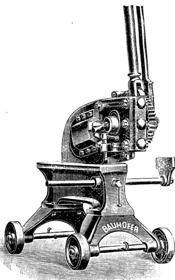
Blech- und Profilschere mit direktem und übersetztem Exzentriehel, gleich vorteilhaft verwendbar für schwere und leichte Arbeiten.
