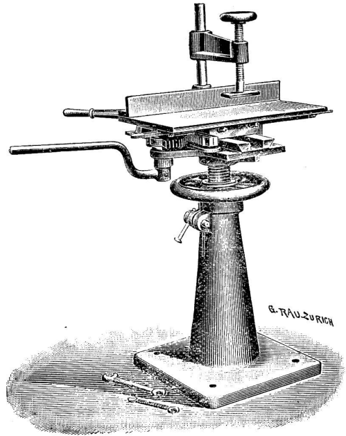
Bohrstander
