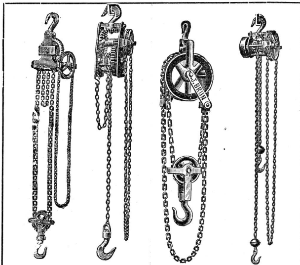
Schraubenflaschenzüge, Brun's Pat. 14539, sowie Schnellflaschenzüge, Differentialflaschenzüge, Winden, Wellenböcke liefert prompt und billig 90sb Ketten- u. Hebezeugfabrik J. Brun, Nebikon (Luz.)
