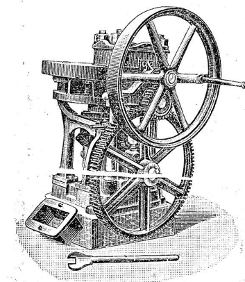
Excenterpresse
