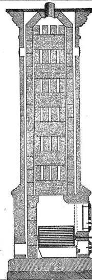
PATENT-OFEN MIT SUTER-EINBAU- QUELSCHOFTE. POLE SUTER-BREVETÉ (S. G. D. G.) COUPES TRANSVERSALES.
