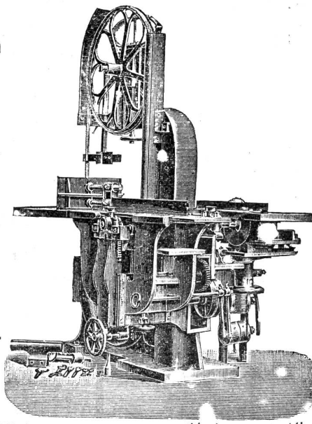
Universalmaschine solidester Konstruktion.
