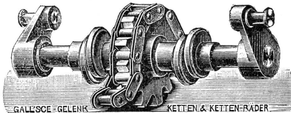
GALL'SCHE GELENK KETTEN- u. KETTEN-RÄDER
