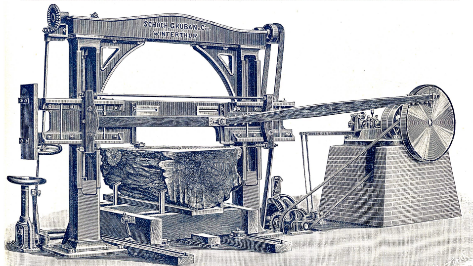
Patent-Horizontalgatter mit einem Vorschub bis zu drei Meter per Minute. Patent Doppelsägerahmen. Scieries horizontales brevetées. Aménage jusqu'à trois mètres par minute. Châssis breveté pour deux lames.
