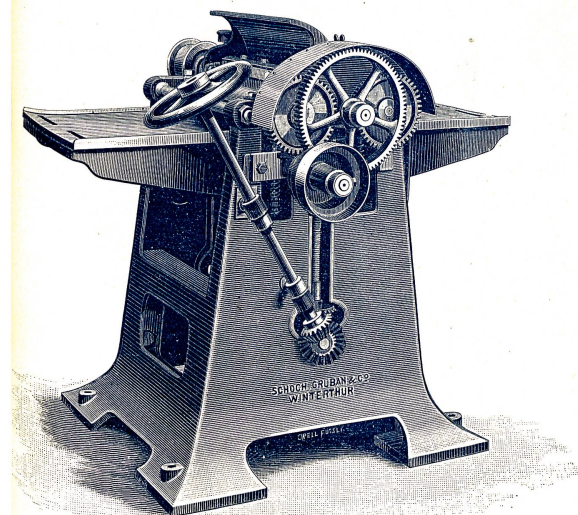
Hobelmaschinen aller Modelle und Grössen. Machines à raboter de toute grandeur.
