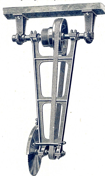
Pendelsägen.
