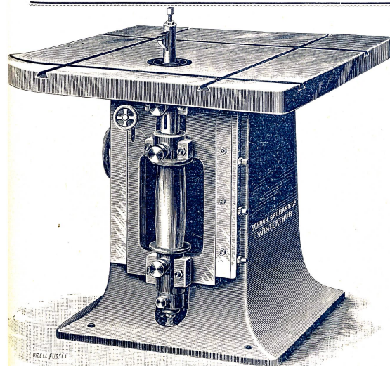
Vertical Kehl-(Frais-)Maschinen mit und ohne amerikanischen Zapfenschlitten.
