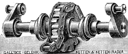
GALL'SCHE GELENK KETTEN &amp; KETTEN-RÄDER
