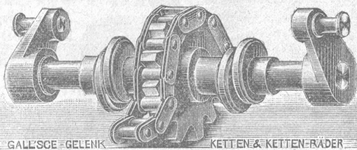
GALL'SCHE GELENK
