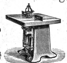
Fräs-Maschine.
