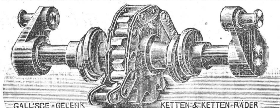
GALL'SCHE GELENK
