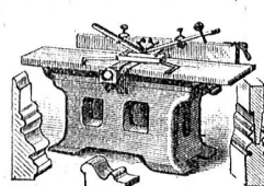
Univers.-Abricht-, Füge- und Kehlmachine.
