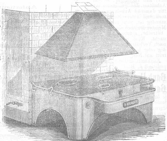
Schmiede-Esse für ein und zwei Feuer, vorzüglich regulirbarem, Kohlen sparendem Feuer, grossem Wasserbehälter und ausziehbarem Träger.
