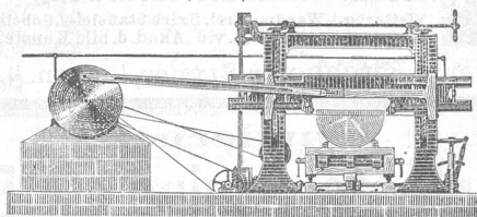
Horizontal-Sägegatter
