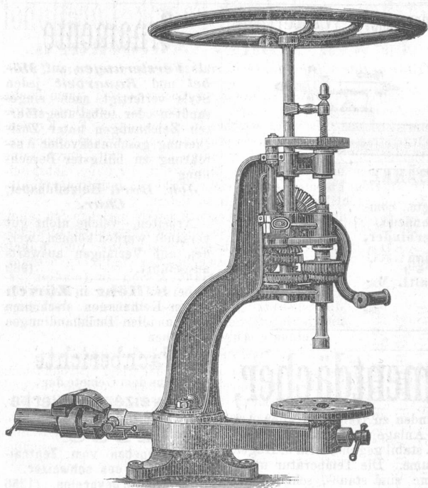
Tischkrieger-Bohrmaschine für Hand- und Kraftbetrieb mit drehbarem, horizontal verschiebbarem Tisch und Parallelschraubstock, zweifacher Uebersehung, zwei Geschwindigkeiten und Selbstschaltung.
